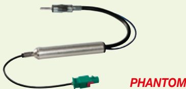
08541 FAKRA → DIN Packed 1 pc. 085413 Packed 20 pcs.
